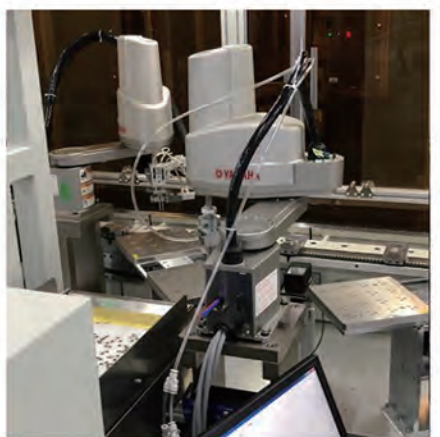
心脏手术器械组装
