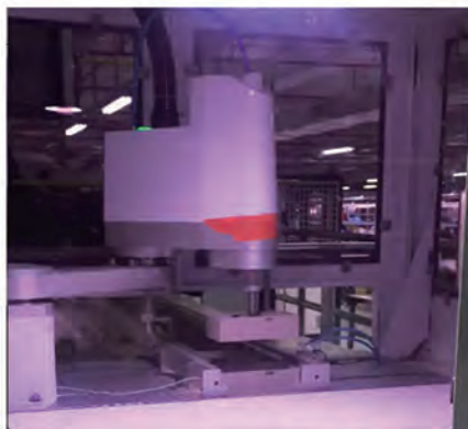
视觉引导纸盒包装
