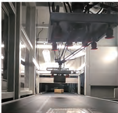
Delta机械手包裹分拣
